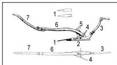
Arado de madera adquirido en Montehermoso en 1945 (Museo Nacional de Antropología). Según J. L. Mingote 1. Reja; 2. Dental; 3. Esteva; 4. Orejeras; 5. Telería; 6. Cama; 7. Timón
